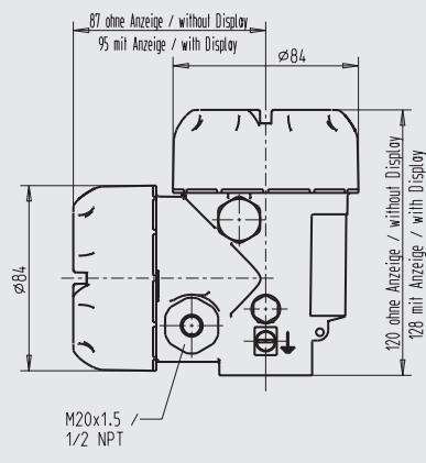
Caja de dos cámaras en aluminio
