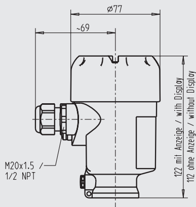
Caja de una cámara, acero inoxidable embutido
