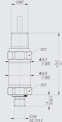
Con salida de cable 1/2 NPT conduit
