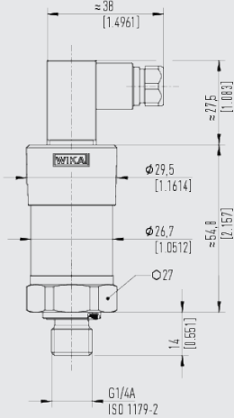
Con conector angular DIN EN 175301-803 C
